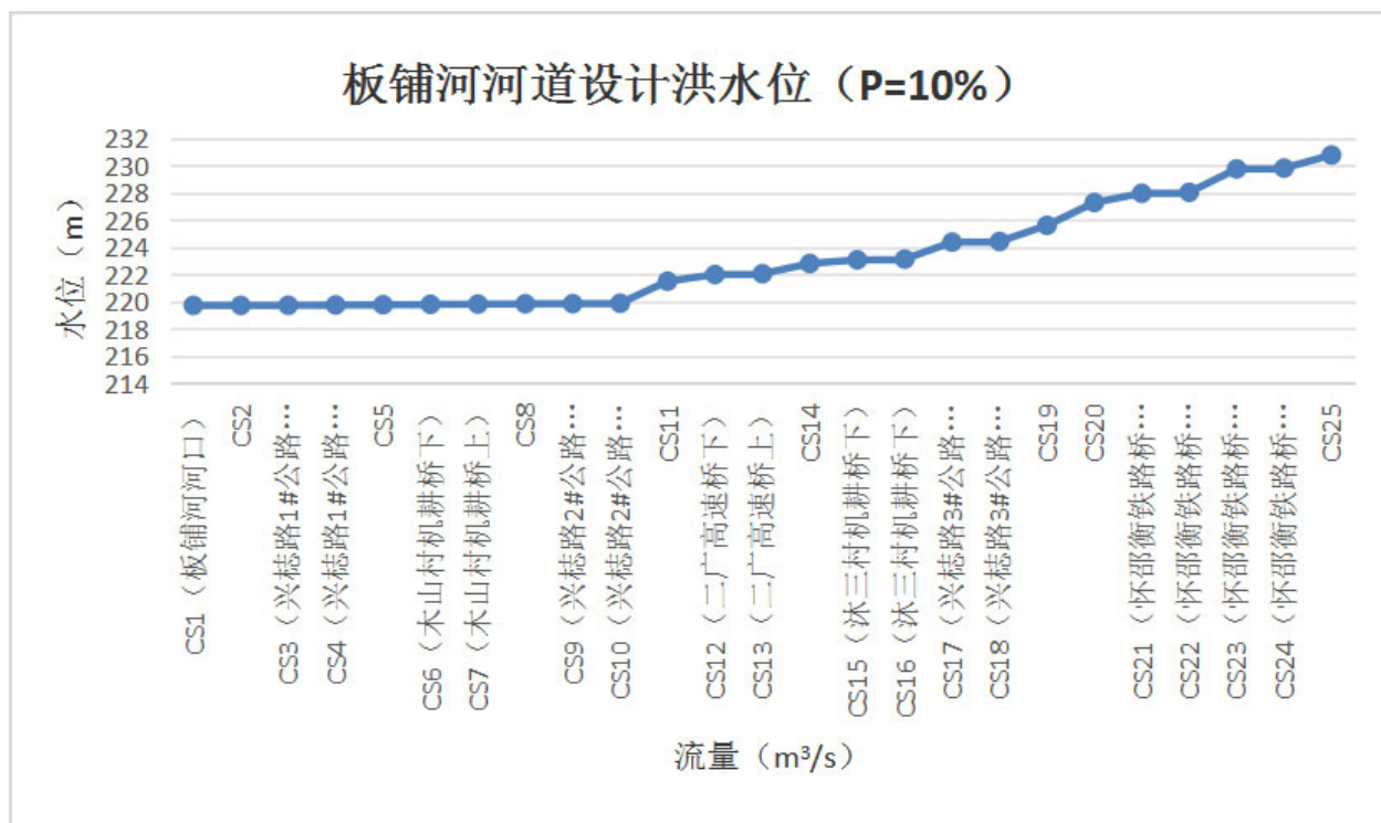
图 4.3 邵阳市北塔区板铺河河道洪水位标图 (P=10%)
