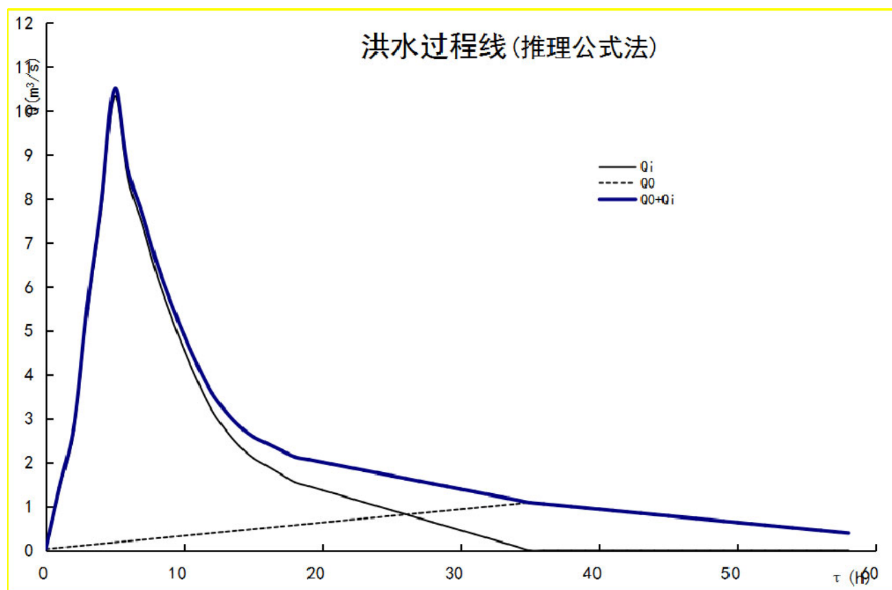
图 4.1 板铺河流域设计洪水过程线
