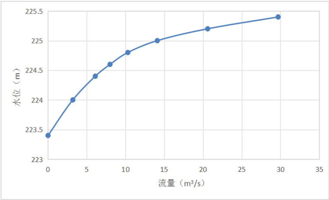
图 4.2 兴桔路 3#公路桥下游水位-流量关系曲线
